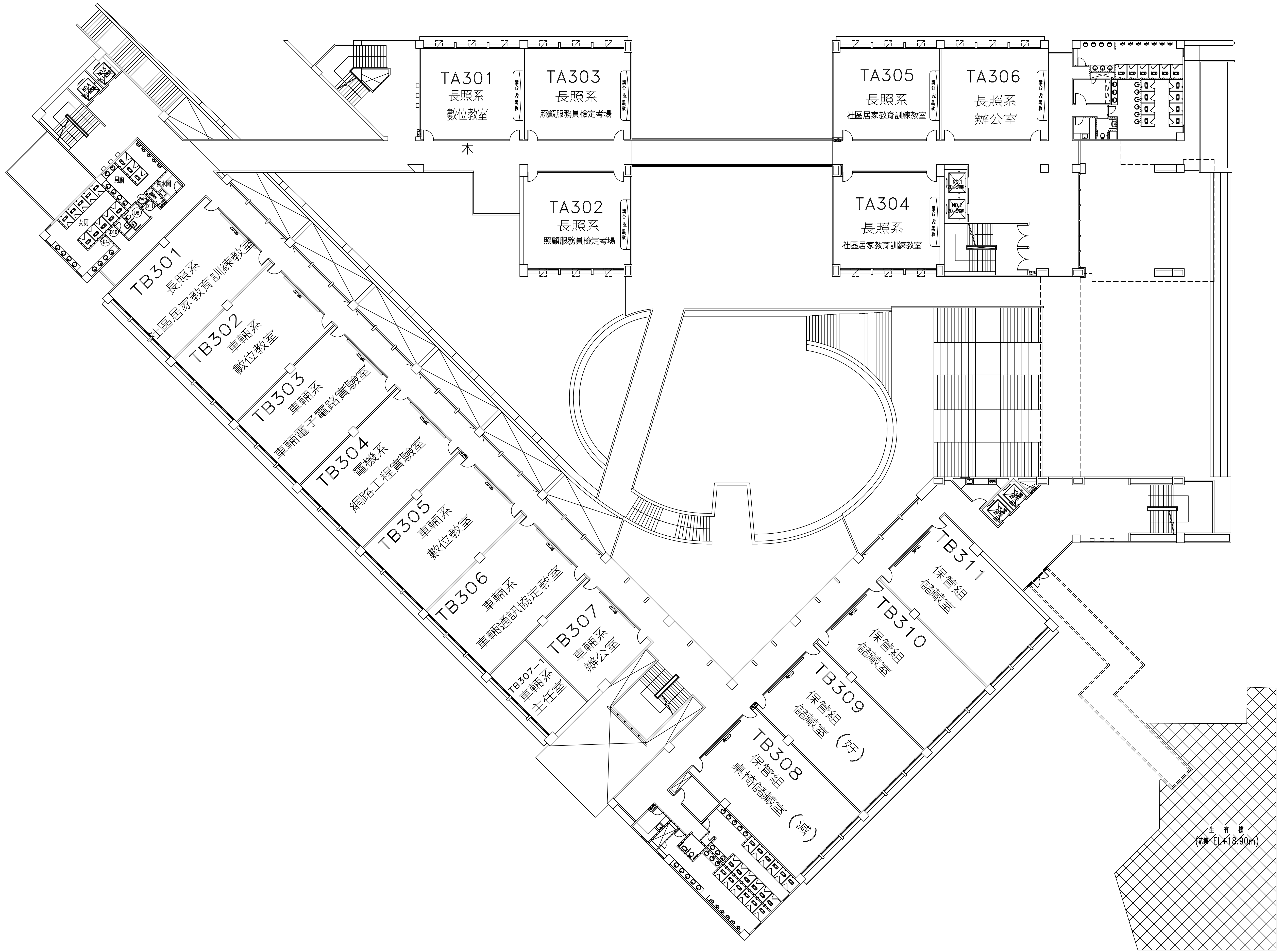
花明樓參層平面圖
