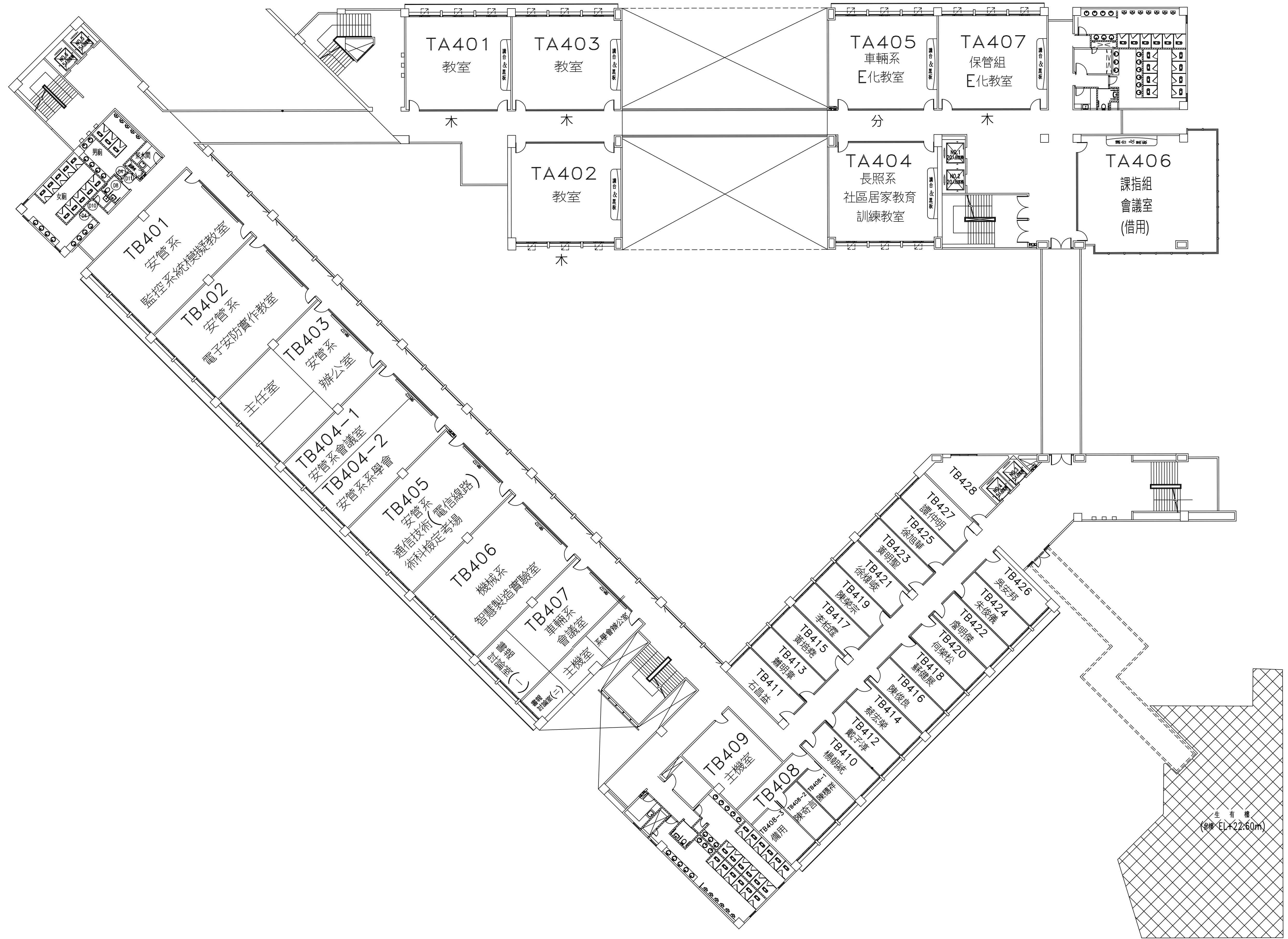
花明樓肆層平面圖
